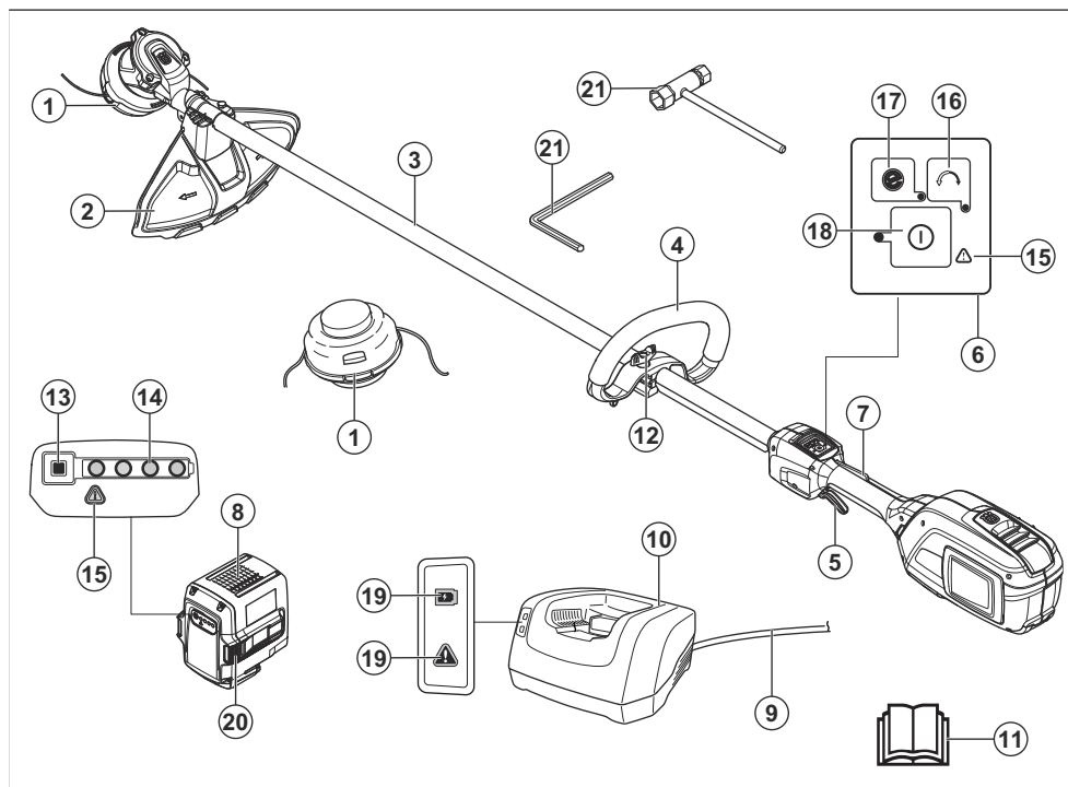
1. Kosilna glava
